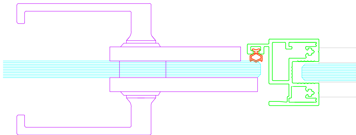
CAM KAPI DETAYI
