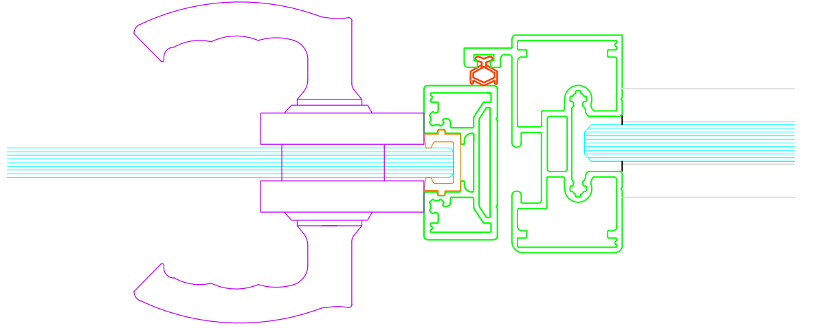
ALÜMİNYUM KENARLI CAM KAPI DETAYI
