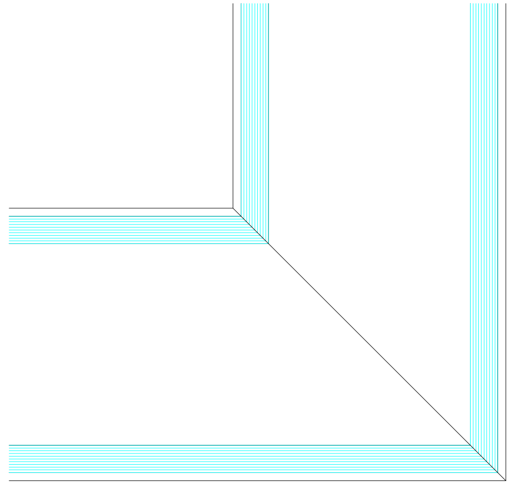
ÇİFT CAM CAMA KÖŞE BİRLEŞİM DETAYI
